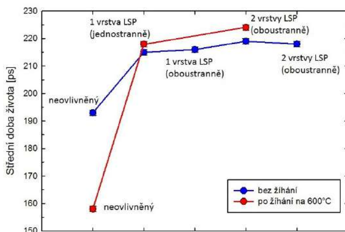
Graf3: Měření doby života pozitronů na vzorku bez ovlivnění, s 1 vrstvou LSP a se 2 vrstvami LSP (modré hodnoty), totéž pak pro vzorky, které byly před ovlivnění vyžehány na 600 °C po dobu 1h (červené hodnoty).
