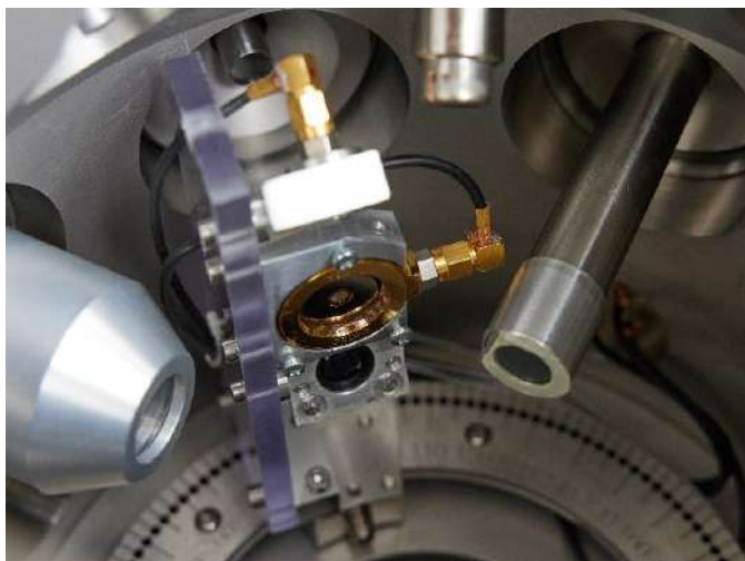
Obr. 1. Komora mikrosvazku s držákem vzorků a vnitřní uspořádání detektorů, kamer a mikroskopu.
