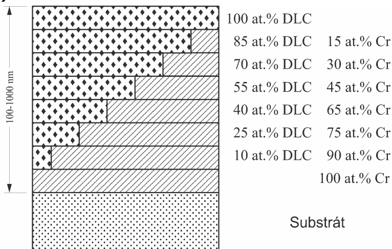
Obr. 1 A) Ukázka multivrstvých struktur CrN / \nabla Cr:DLC, TiO 2 / \nabla Ti:DLC a TiN / \nabla Ti:DLC. B) Hybridní systémy pro přípravu dopovaných vrstev. Schéma depozičního systému pulzní laserové depozice s magnetronovým naprašováním: 1 - Substrát, 2 - Grafitický terč, 3 - Laserový svazek, 4 - Magnetron, 5 - Záslepka magnetronu, 6 - Rotace, 7 - RF elektroda, 8 - Vakuová měřky, 9 - Turbomolekulární pumpa, 10 - Průtok plynu (Ar / N / O)
