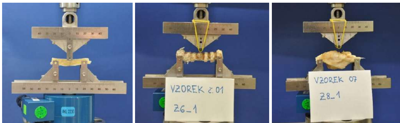
Obr. 1 Průběh zatěžování na speciálním přípravku pro tříbodový ohyb, vlevo – intaktní žebro, uprostřed – žebro fixované, vpravo – žebro nefixované
