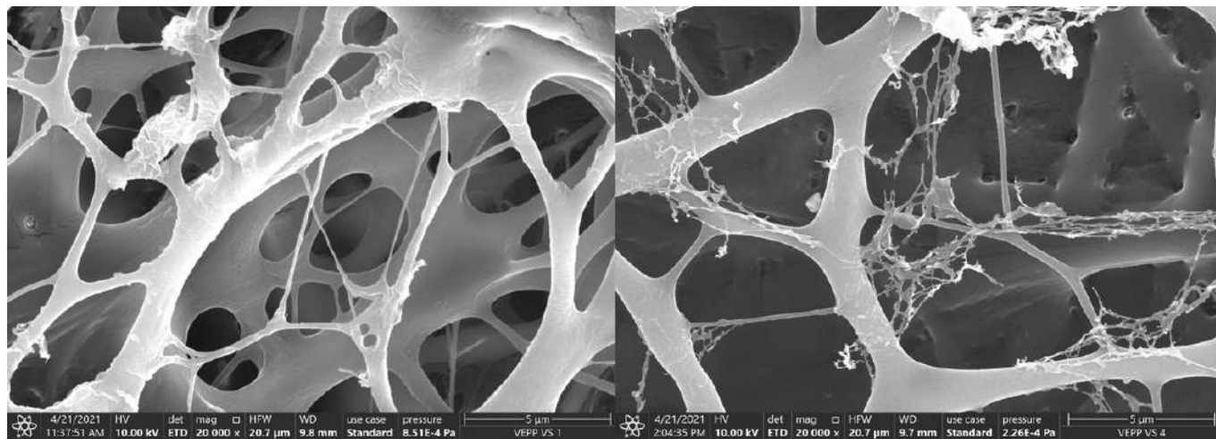
Obr. 1 Na snímku ze SEM vlevo je vrstva zvlákněná z roztoku PBS/etanol (20 000x). Vpravo je vzorek připravený z roztoku kyseliny octové modifikovaný glycerinem (20 000x).
